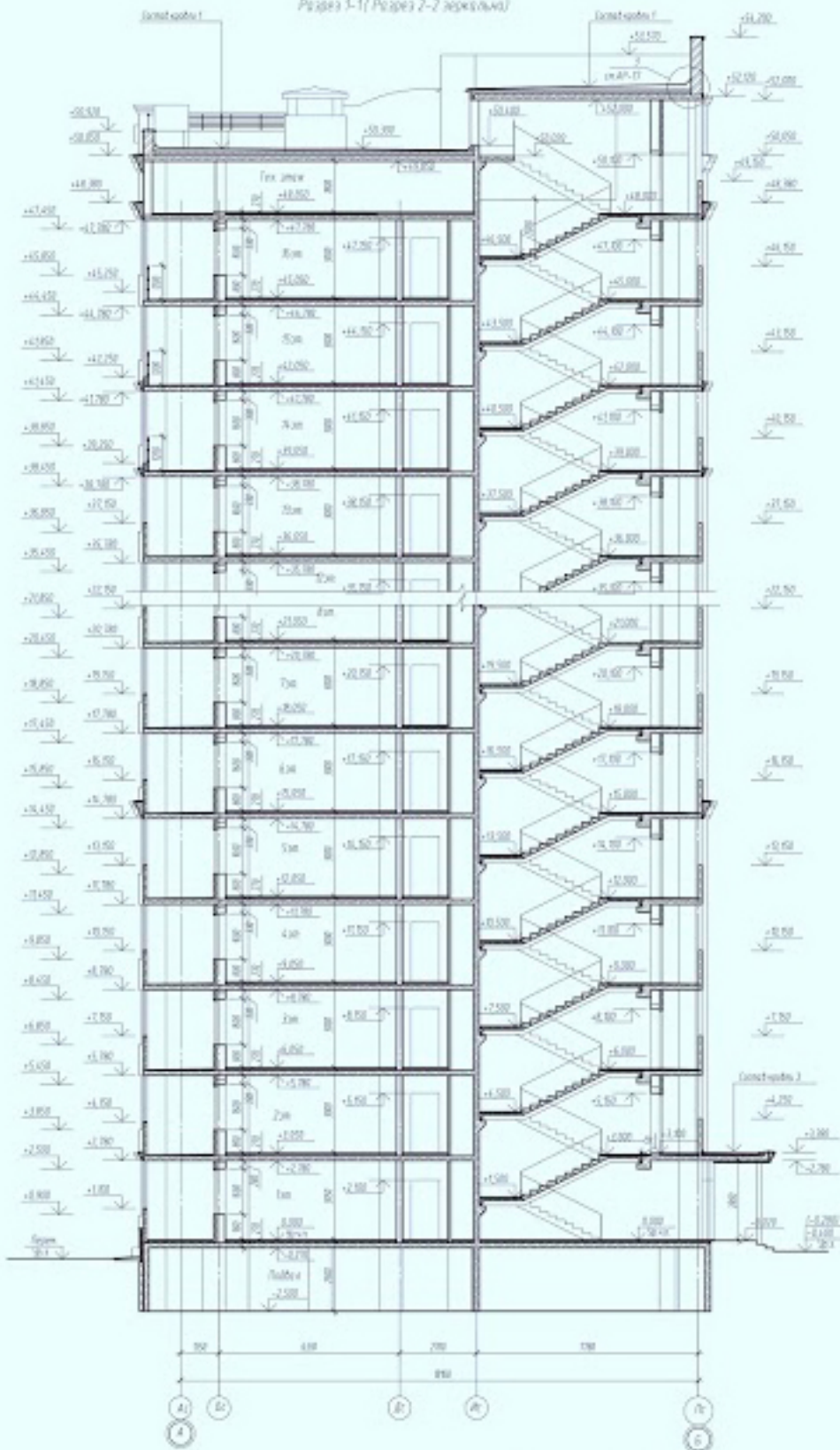
Разрез 1-1 (Разрез 2 зеркально)
